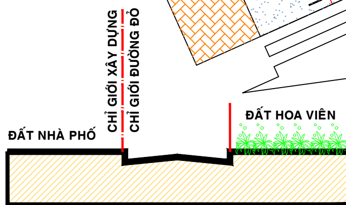
MẶT CẮT 2 - 2
