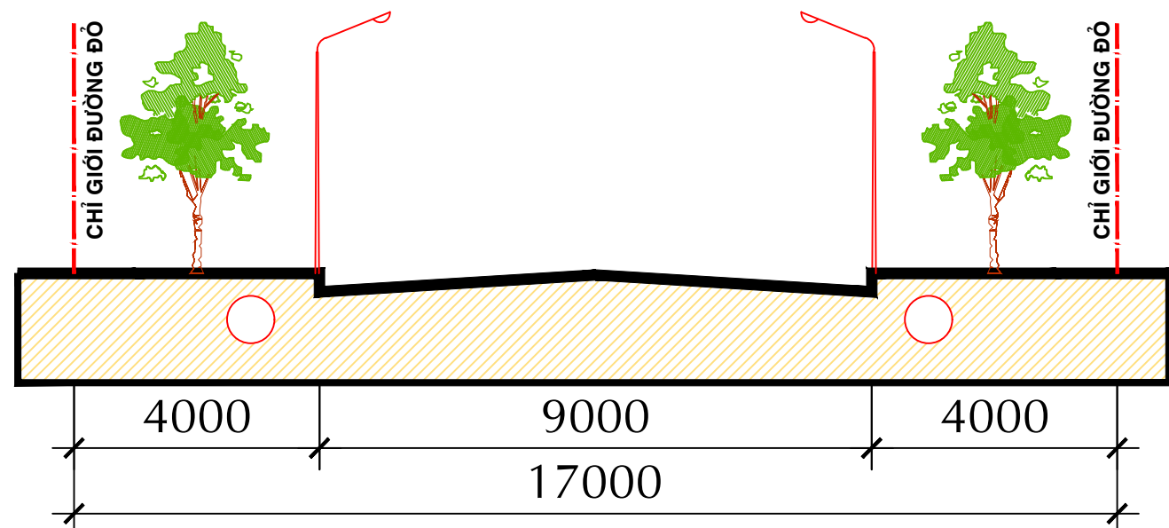
MẶT CẮT 1 - 1
